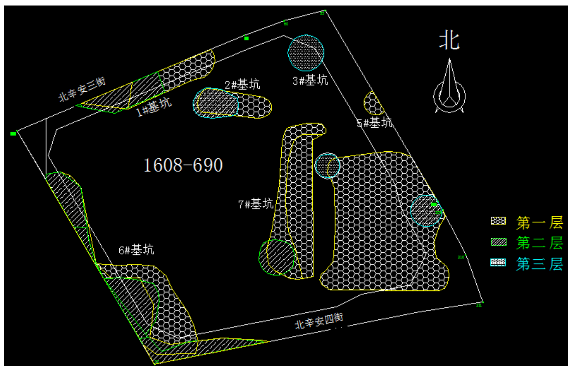
图 15.2-1 690 地块污染土分层图
