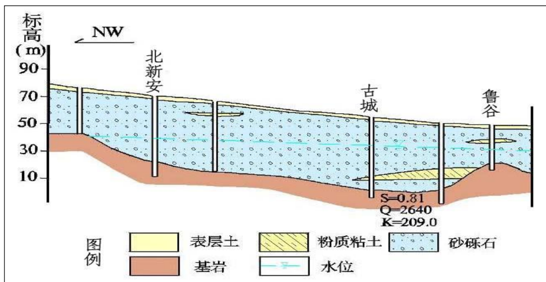
图 1.3-6 石景山水屯-马家堡 (A-A') 地层剖面图
