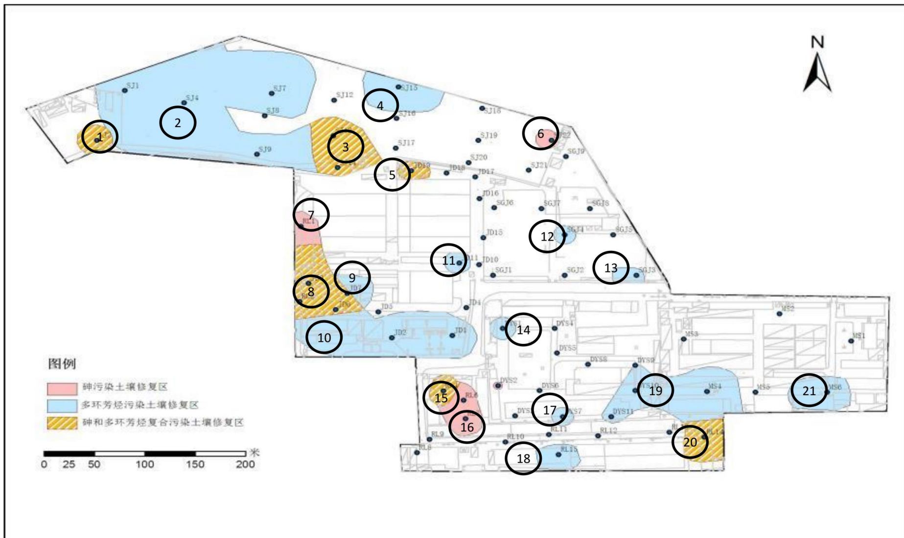
图 1.4-2 污染土壤第二层(1-2m)修复范围示意图
