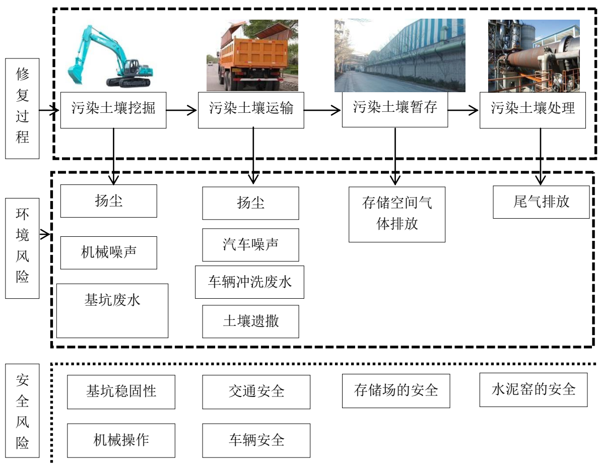
图 8.1-1 污染土壤修复过程中的污染源分析
